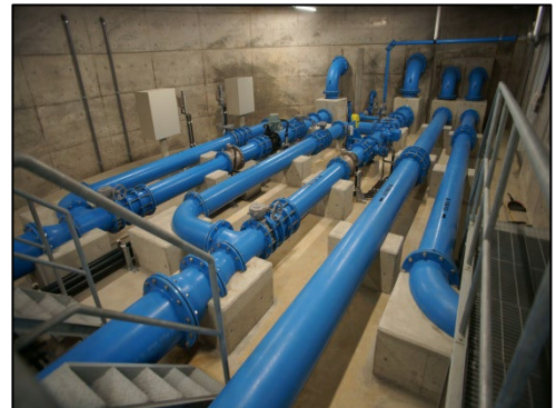
配水塔内配管 P L P φ350~φ450
